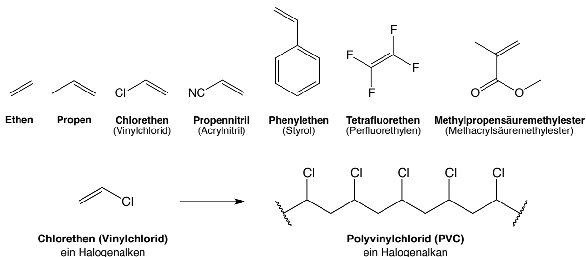
Abbildung 12: Formeln und Namen einiger gängiger Monomere, welche Kunststoffe bilden können (oben) sowie die Polymerisation von Chlorethen zu PVC (unten)
