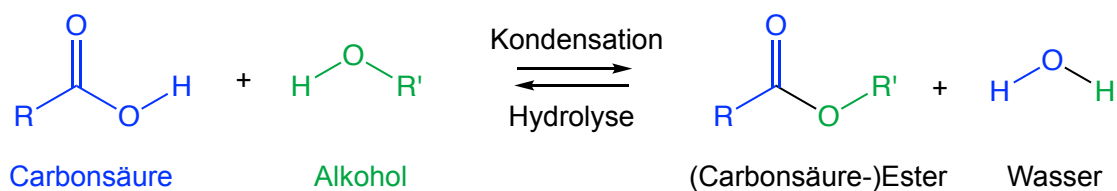
Abbildung 5: Reaktionsschema zur Kondensation und Hydrolyse am Beispiel der Veresterung und der Esterhydrolyse; R und R' sind Alkylreste.
