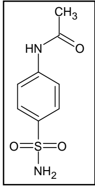
p-Acetamidobenzen-sulfonamid und
