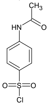
p-Acetamidobenzensulfonylchlorid:
