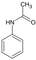
Acetanilid:
