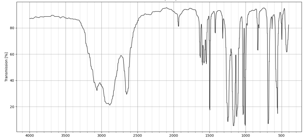
p-Acetamidobenzensulfonylchlorid:
